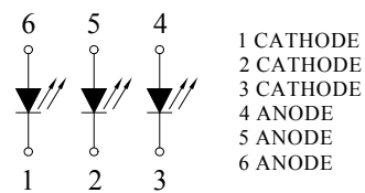
Polarity
