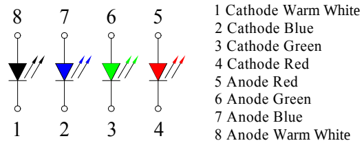
Polarity
